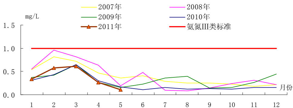
图五 太湖氨氮平均浓度变化趋势
