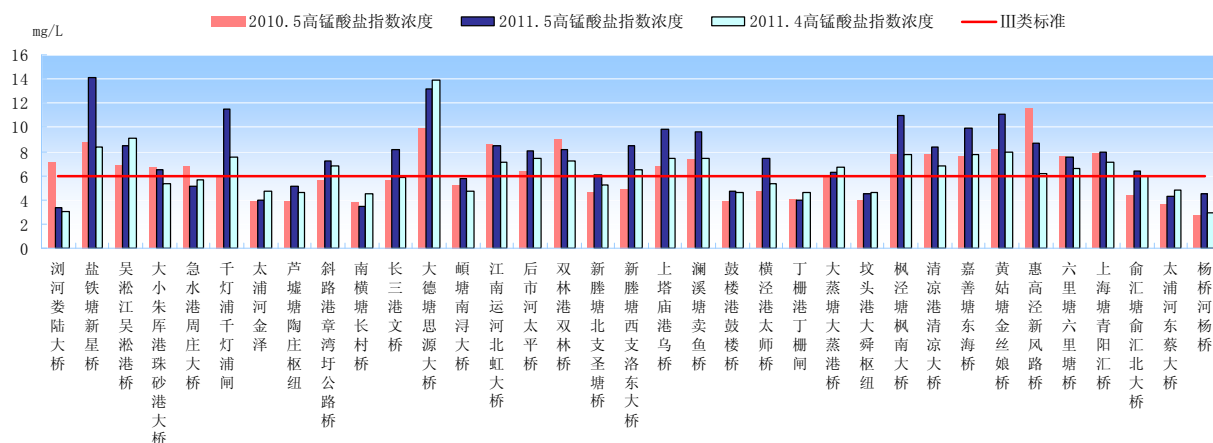
图二 省界河流高锰酸盐指数浓度
