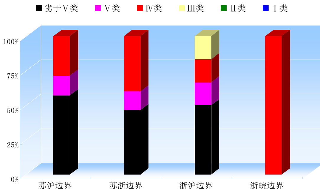
图一 太湖流域省界河流水质类别比例
