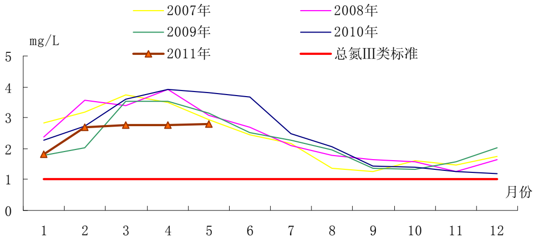
图七 太湖总氮平均浓度变化趋势
